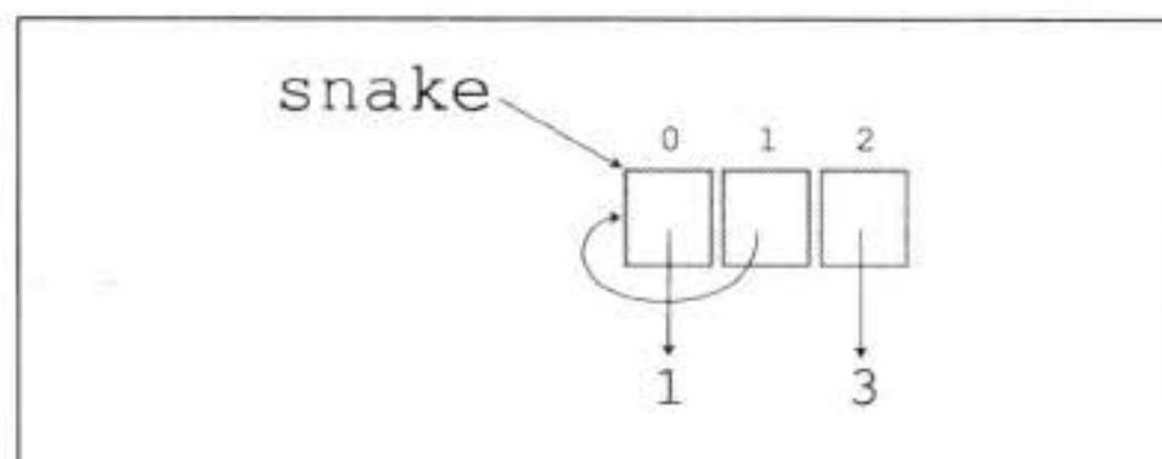
图 7-2 一个自引用列表。请注意，第二个元素指向整个列表，而不是第一个元素
