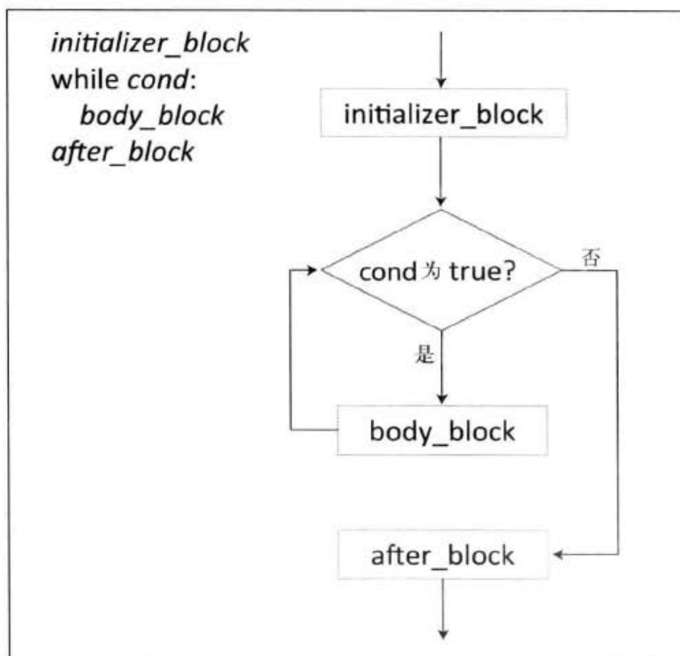
图 4-3 一个描述通用 while 循环的流程图。注意到这里没有专门列出递增语句，因为它位于 body_block 中——通常（但并非总是）位于 body_block 的末尾
